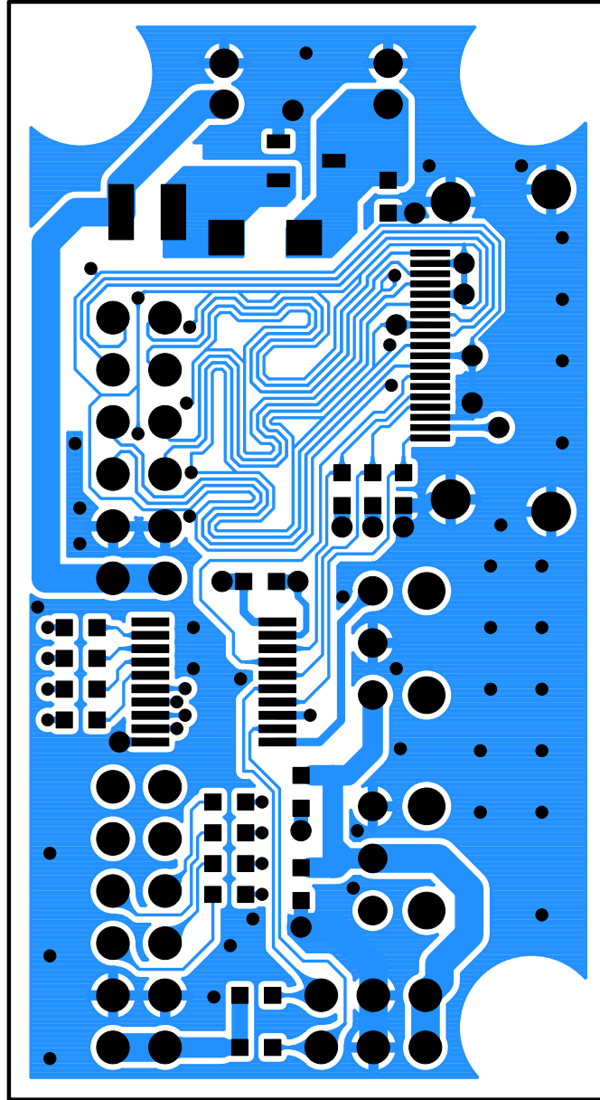
部品面パターン
