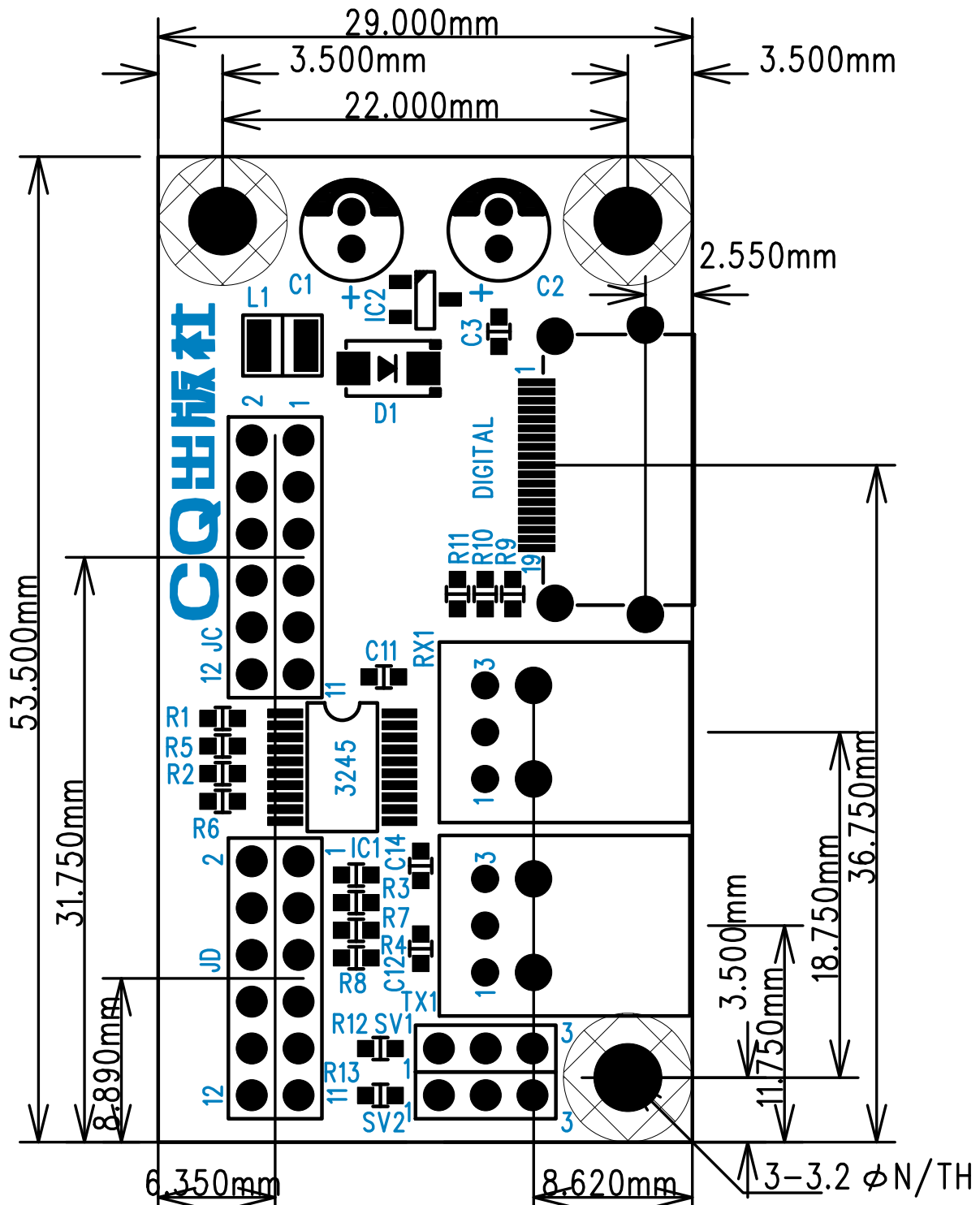
部品面寸法図 部品面シルク ドリル穴図
